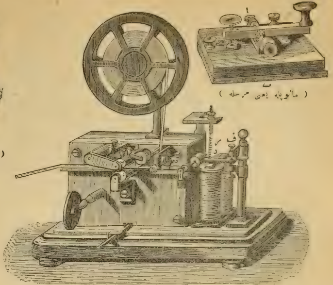
( ایکنه لی مورس ما کنه سی )
